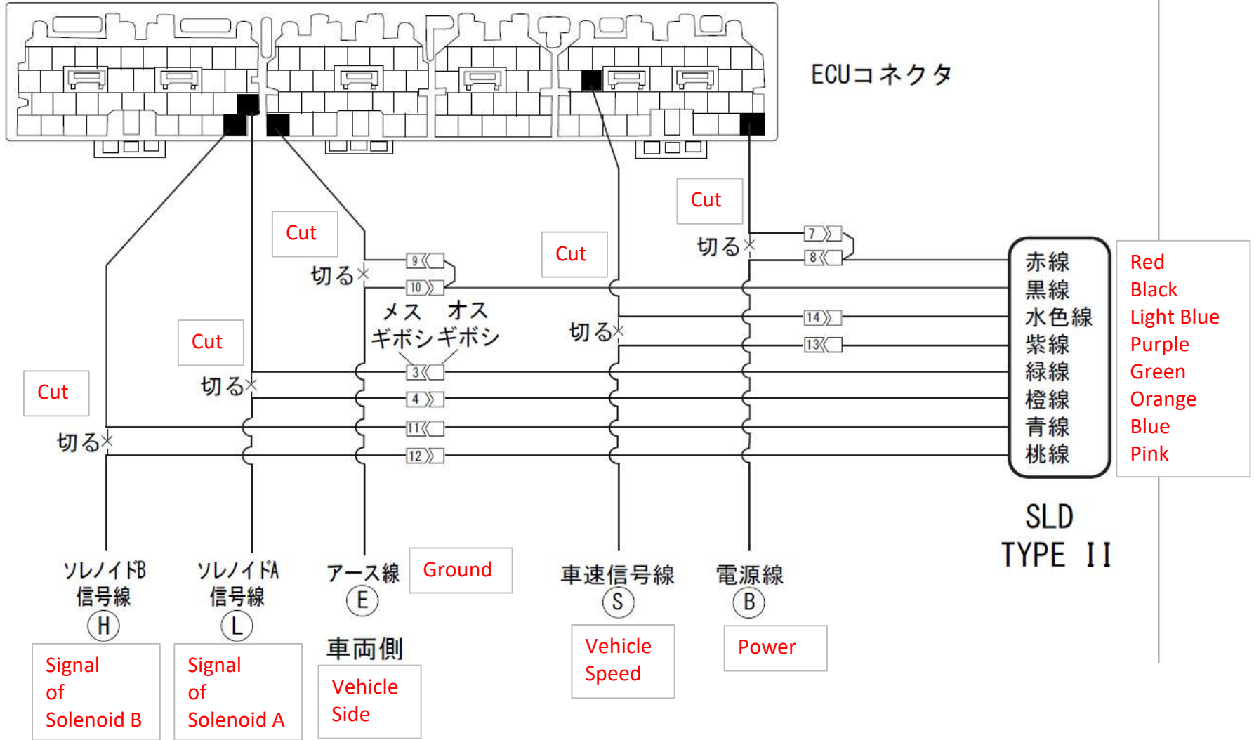
E-1 配線図
